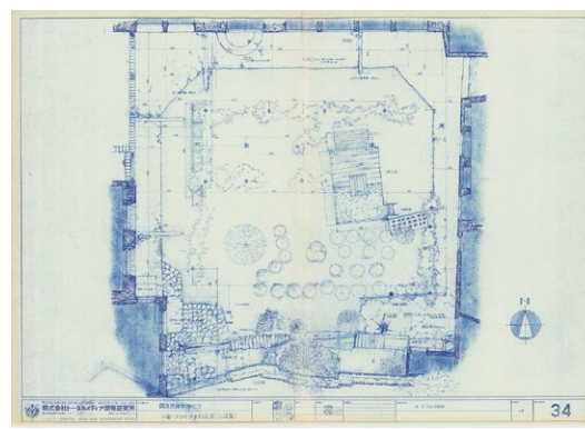
タシュケントの民家(模型縮尺1/10)の青焼き図面 (作成:株式会社トータルメディア開発研究所)
